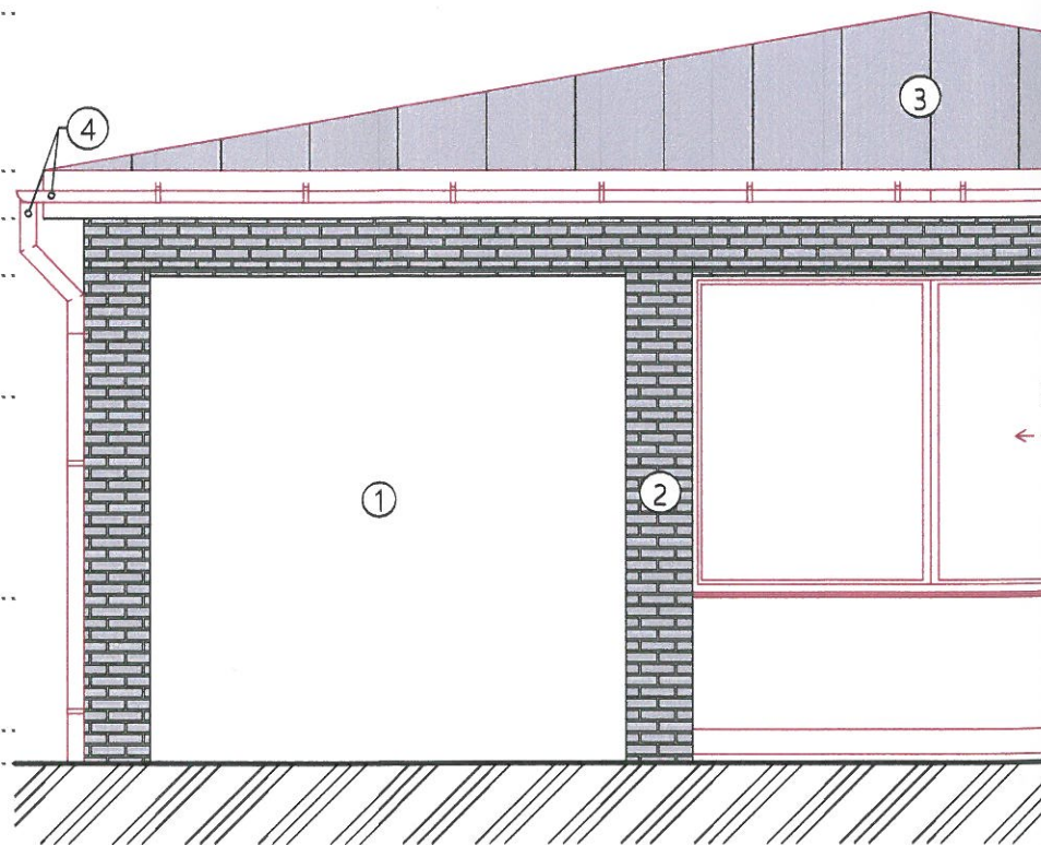
POHLAD VÝCHODNÝ
