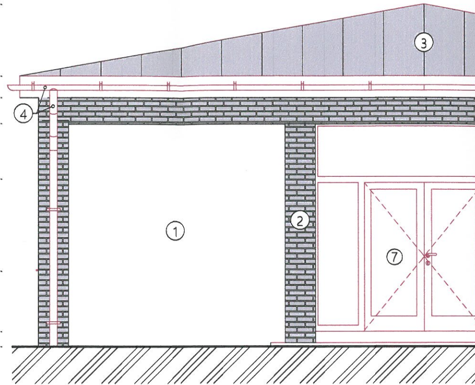
POHLAD JUŽNÝ
